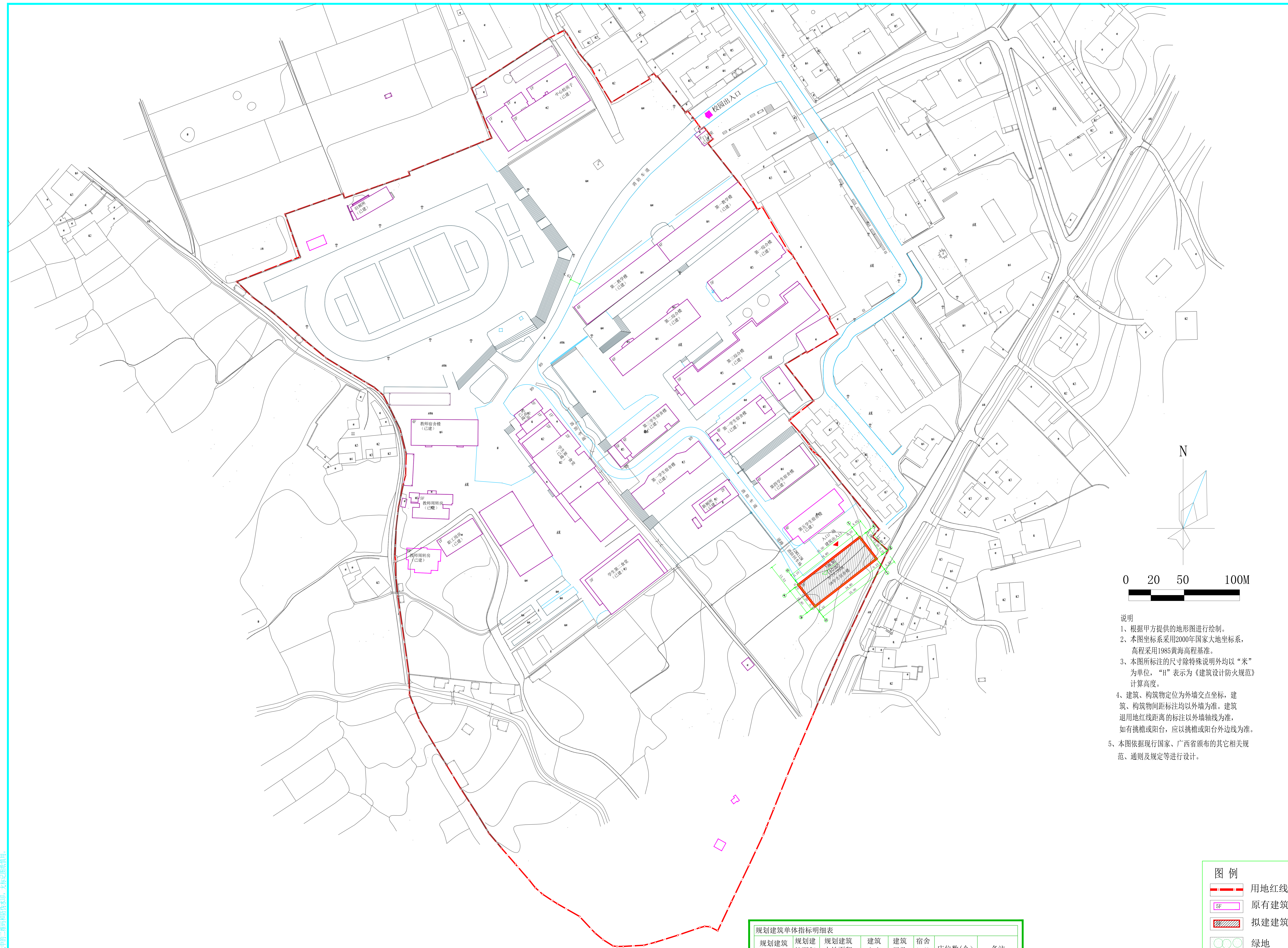
全州县凤凰镇凤凰初中总平面图 1:500
